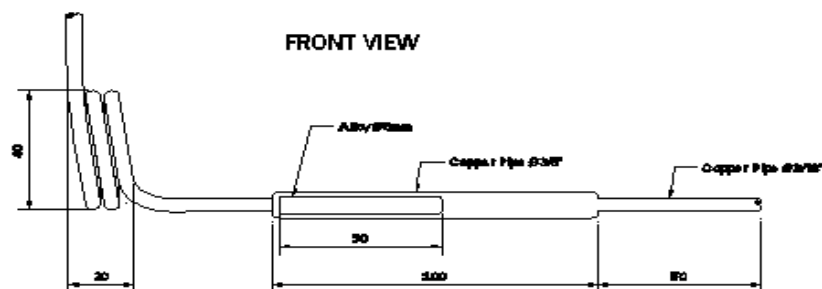
Gambar 1. Desain Pipa katalis spiral HCS
