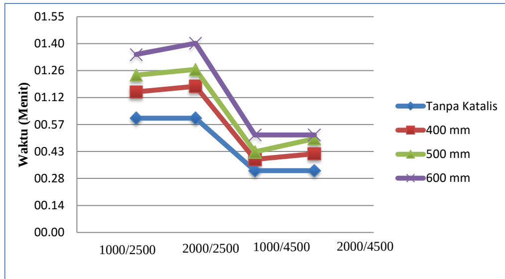
Gambar 3. Waktu penghematan bahan bakar pada kondisi berjalan
