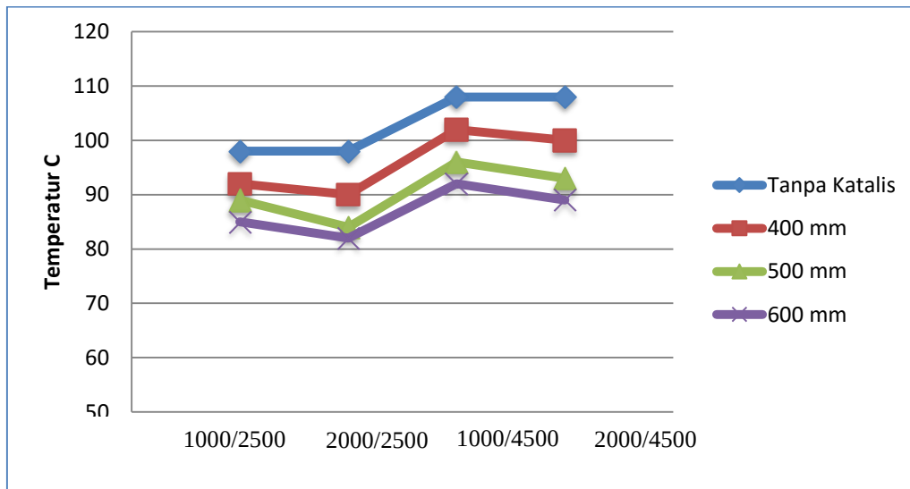
Gambar 3. Grafik pengujian temperatur mesin pada kondisi berjalan
