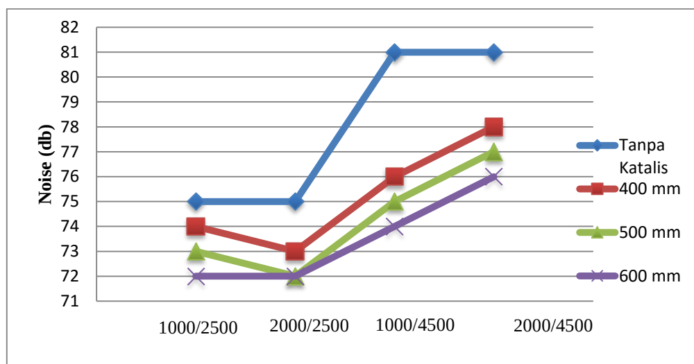
Gambar 4. Hasil uji kebisingan atau noise mesin pada pada kondisi berjalan
