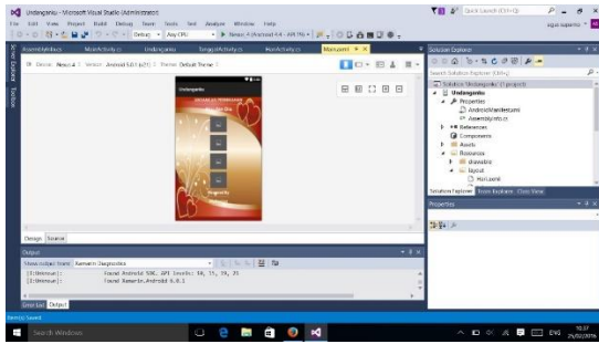
Gambar 14. Tampilan Lengkap
