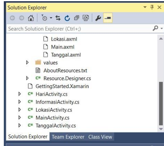
Gambar 12. Semua Activity
