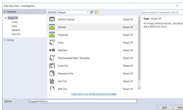
Gambar 11. InformasiActifity
