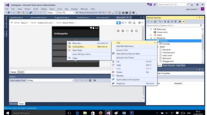
Gambar 13. Menambahkan Background
