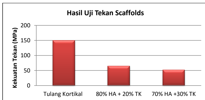
Gambar 5. Hasil uji kekuatan tekan tulang kortikal dan scaffolds
