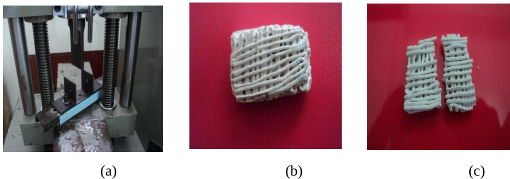
Gambar 4. Uji tekan a) mesin UTM b) Spesimen c) patahan scaffolds
