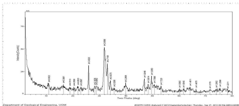
Gambar 3. Hasil uji XRD material scaffolds dengan komposisi 80% TK + 20% HA
